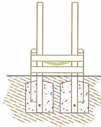
End Elevation
