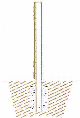
End Elevation
